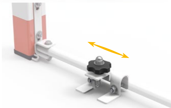
(6) - Pattes d'ancrage amovibles Réf. HB050415
